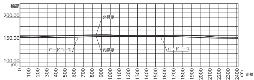
オーバルコース縦断図
